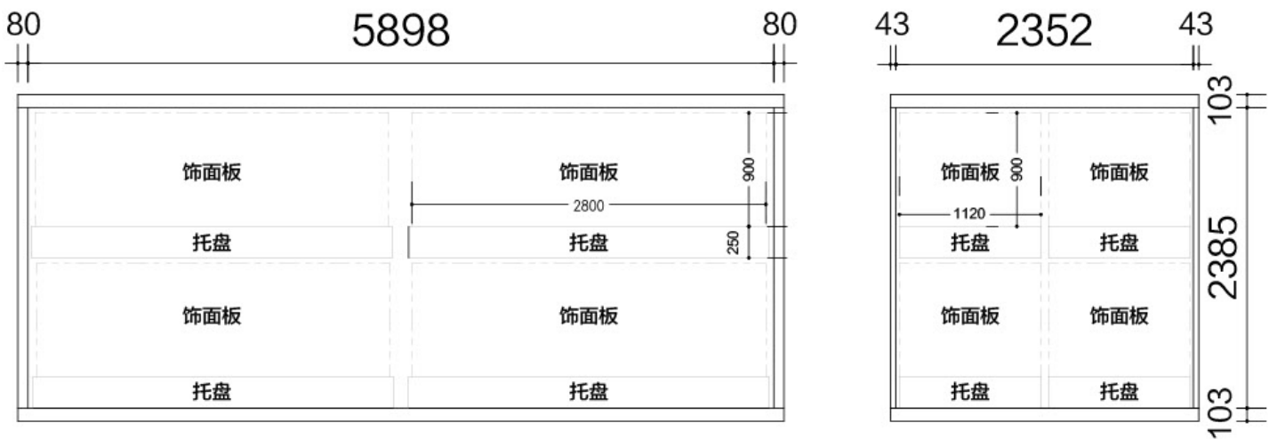
20正常装货货柜尺寸
