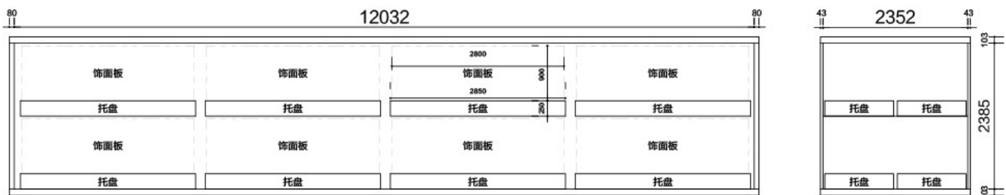
40正常装货货柜尺寸
